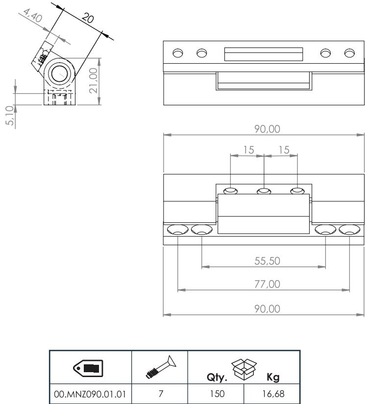
Zinc Door Hinge 90 mm For Adopen Marmara
