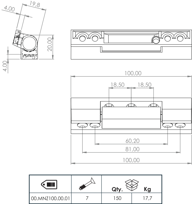
● Zinc Door Hinge 100 mm
