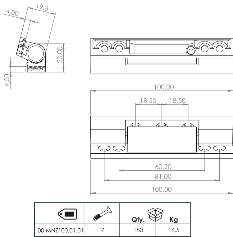
Zinc Door Hinge 100 mm / Economic
