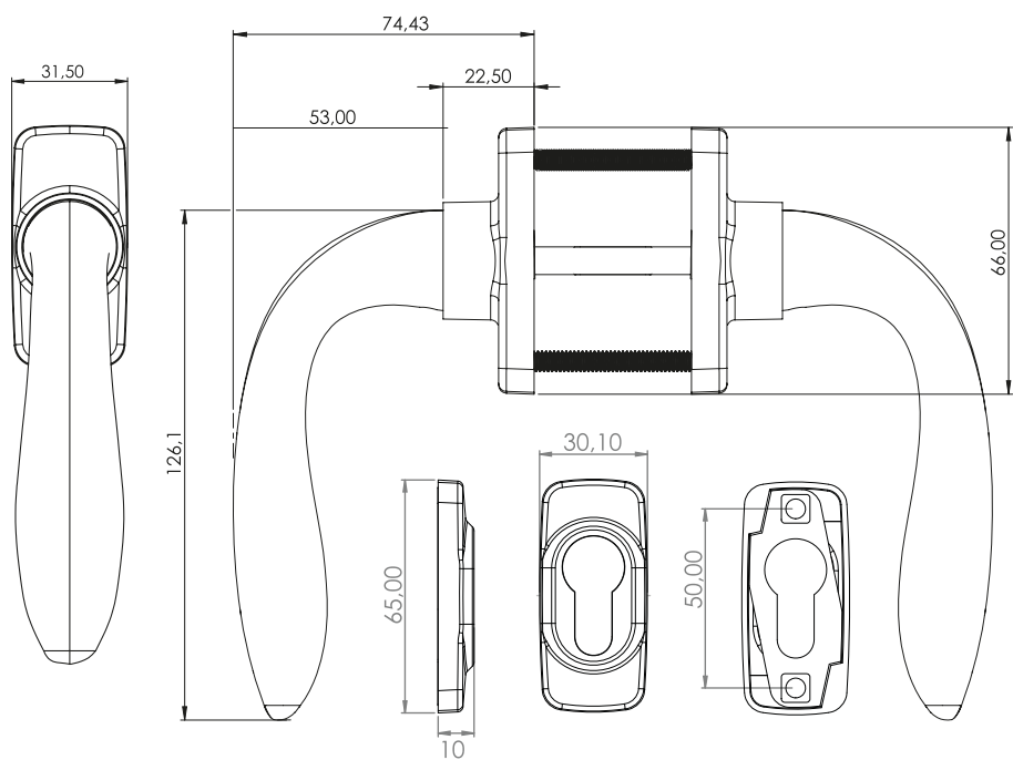
● Ada Aluminium Door Handle
